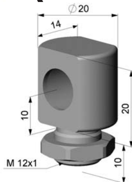
Montagebolzen mit M 12x1-Gewinde justierbar in einer Achse
