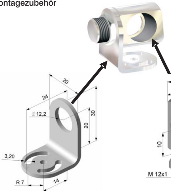
Montagewinkel, justierbar in einer Achse
