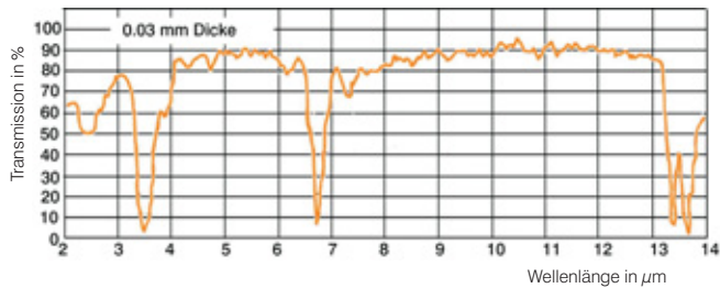
Spektrale Durchlässigkeit von Kunststofffolien aus Polyester
