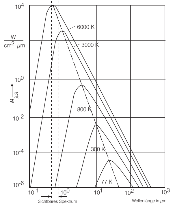
Spektrale spezifische Ausstrahlung M_{\lambda, s} des schwarzen Körpers in Abhängigkeit von der Wellenlänge
