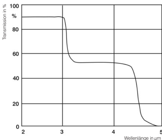
Spektrale Durchlässigkeit von Glas
