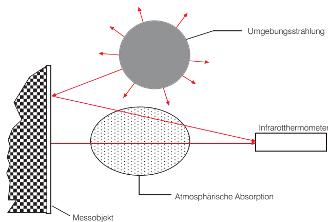
Umgebungsstrahlungskompensation
