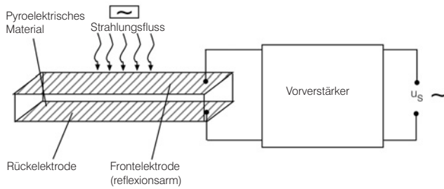
Prinzipieller Aufbau eines pyroelektrischen Detektors
