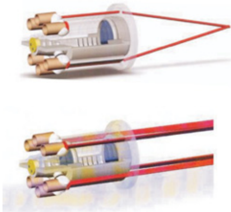
Optomechanischer Aufbau eines modernen Infrarotthermometers
