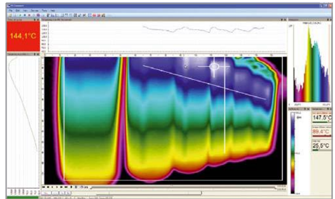
optris PI in Verbindung mit einem Tablet-PC für mobile Anwendungen
