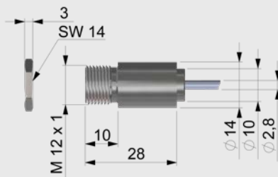
Messkopf
