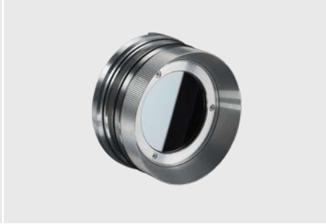
ACCJAFUxx + ACCJAPWPI2xxLW / ACCJAFUxx + ACCJAPWCTLSW Fokussiereinheit mit Schutzfenster für CoolingJacket
