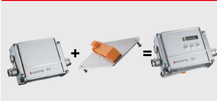
CT Elektronikbox ACCTRAIL Tragschienenmontageplatte Elektronikbox auf Tragschienenmontageplatte
