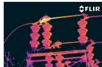
Infrarotbild
